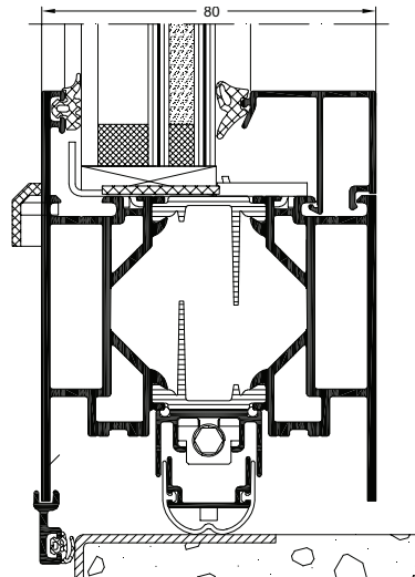
Schüco System ADS 80 FR 30 Vertikalschnitt, Maßstab 1:2
