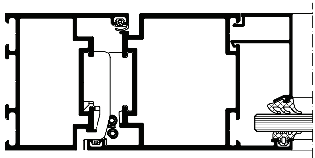
Schüco System ADS 65.NI SP Vertikalschnitt , Maßstab 1:2
